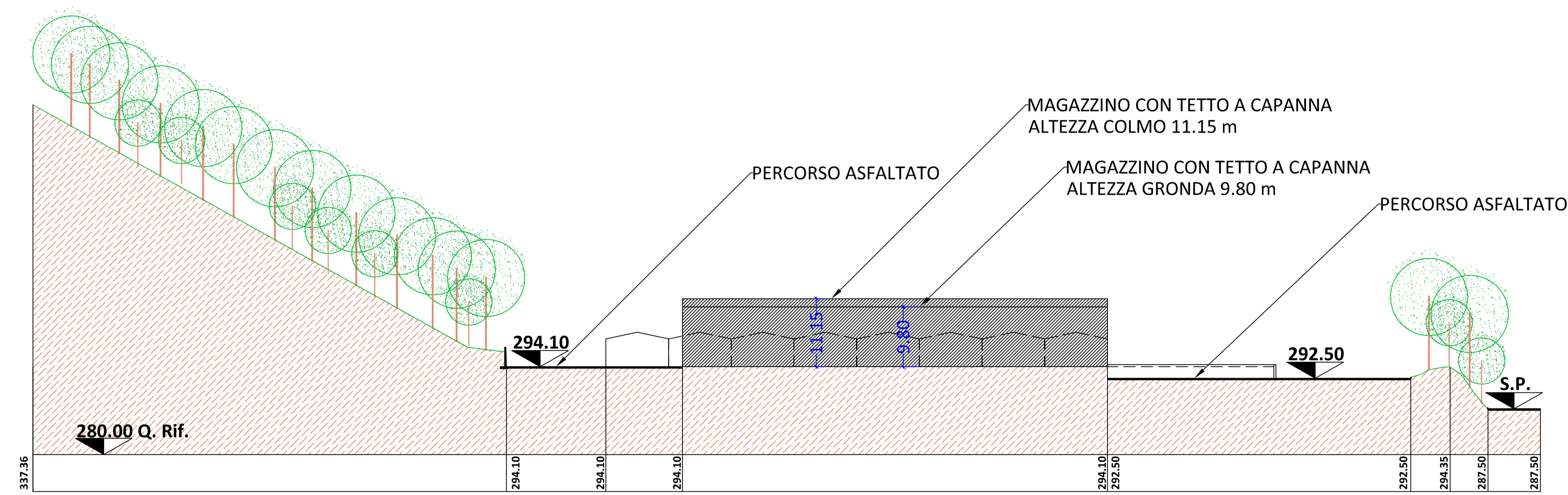
SEZIONE A-A
