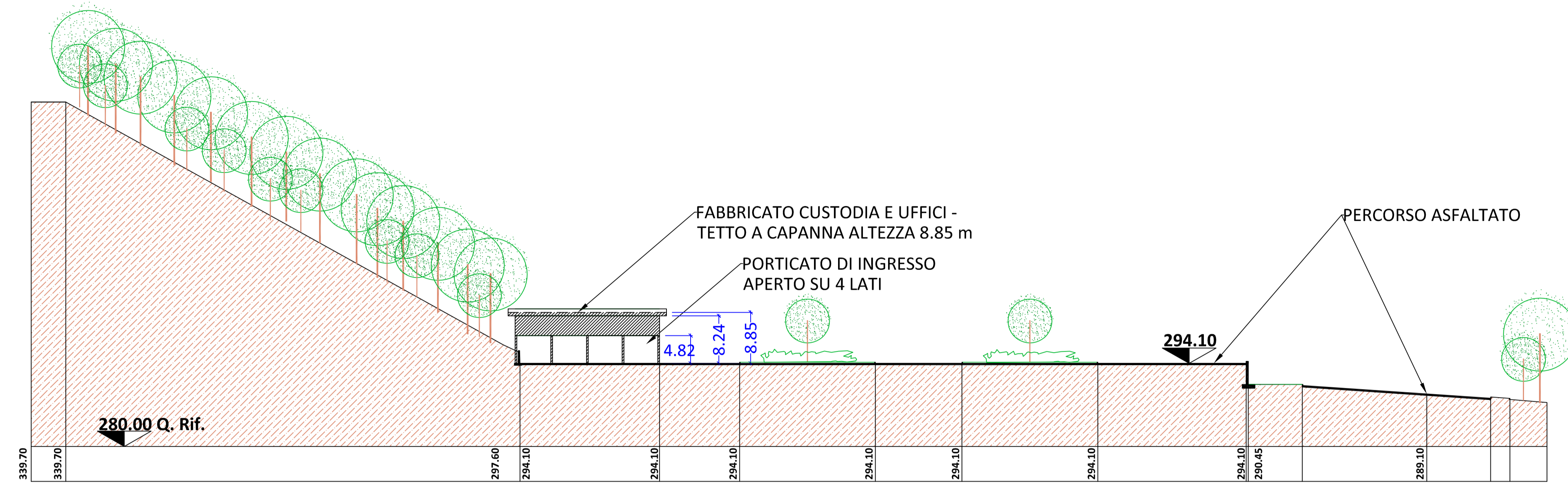
SEZIONE E-E
