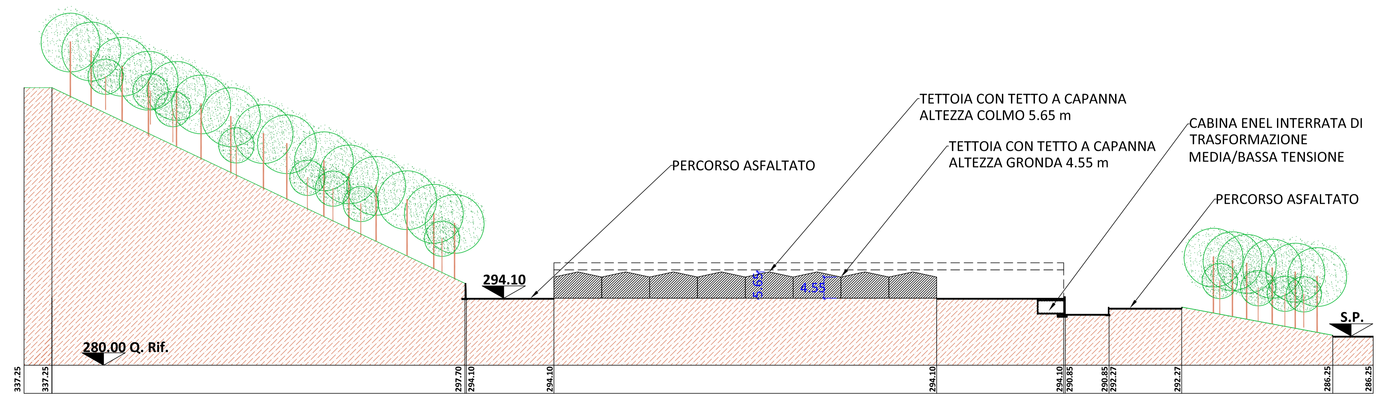
SEZIONE B-B
