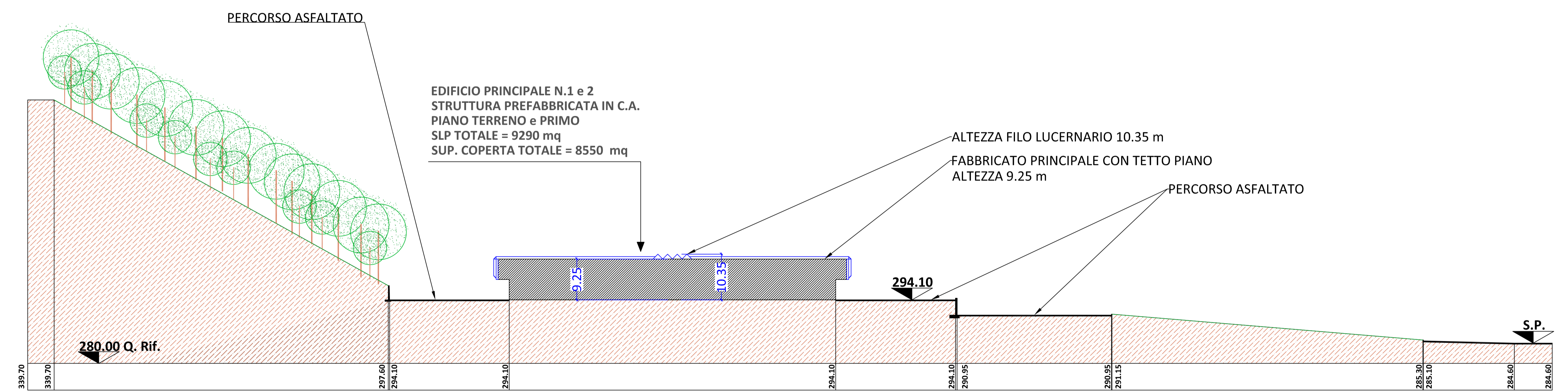
SEZIONE D-D
